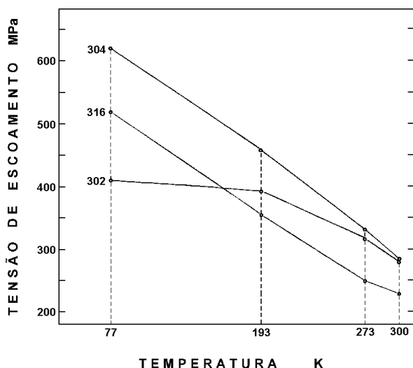
Figura 1 – Influência da Temperatura na Tensão do Escoamento dos Aços.
