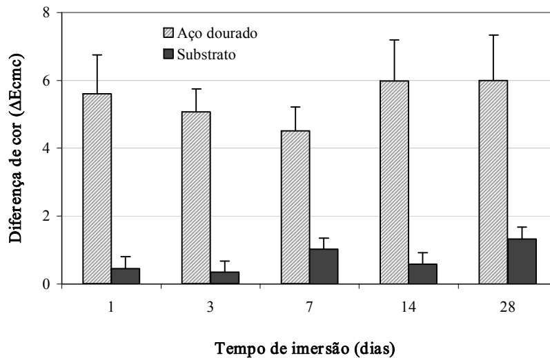
Figura 1 – Valores médios das diferenças de cor obtidas pelas medidas das coordenadas cromáticas (LCh) realizadas nas superfícies das amostras antes e após imersão em chuva ácida simulada pelo tempo indicado.
